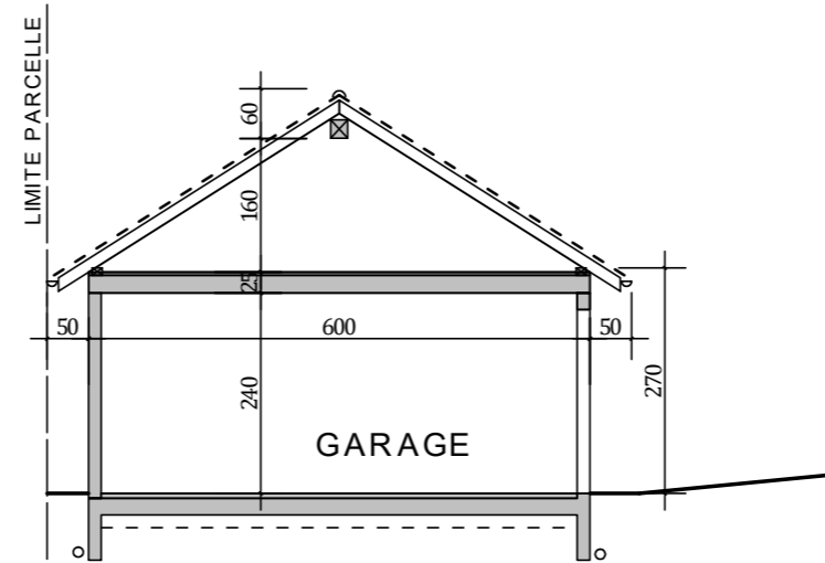
COUPE C-C _ ECH. 1/100
