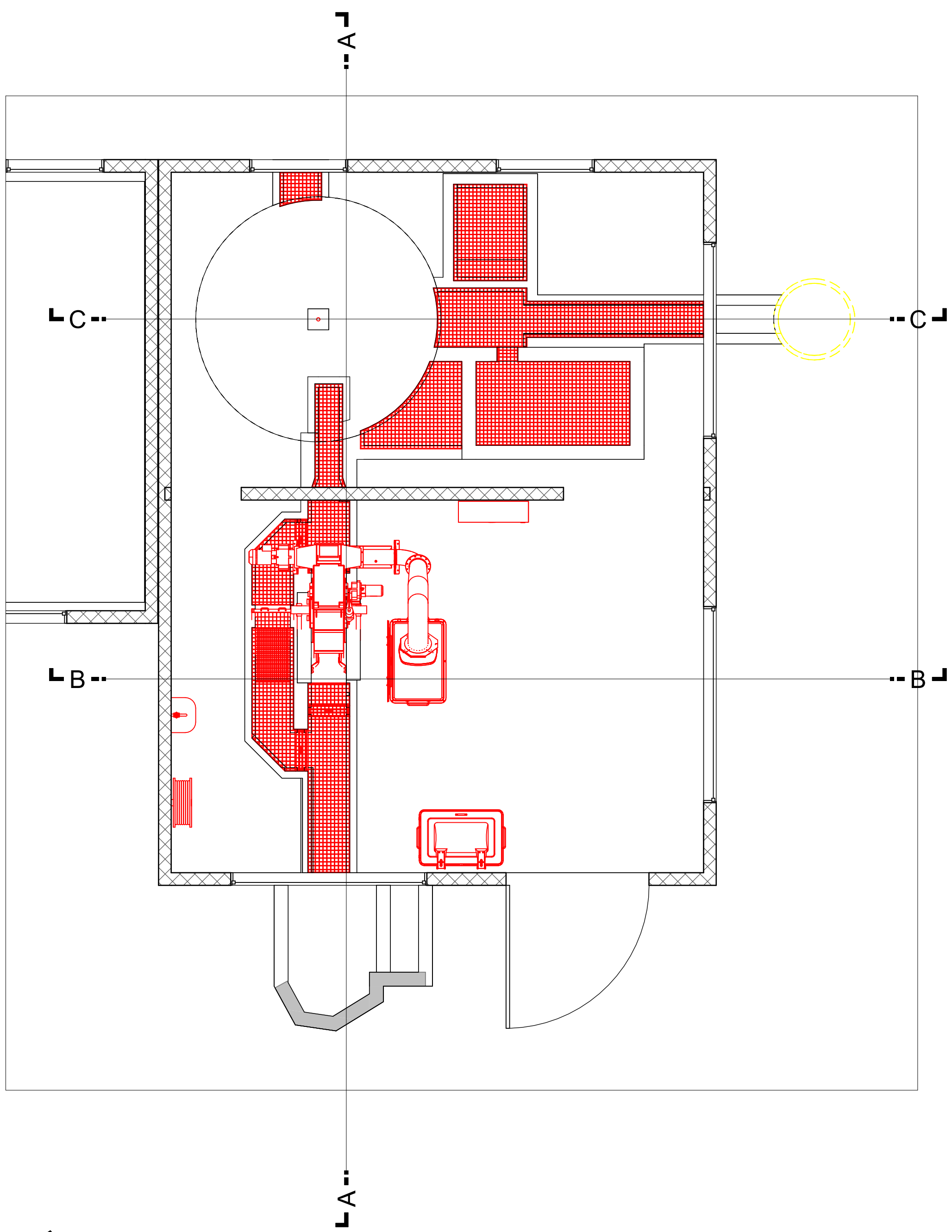
Vue en plan 1 : 50
