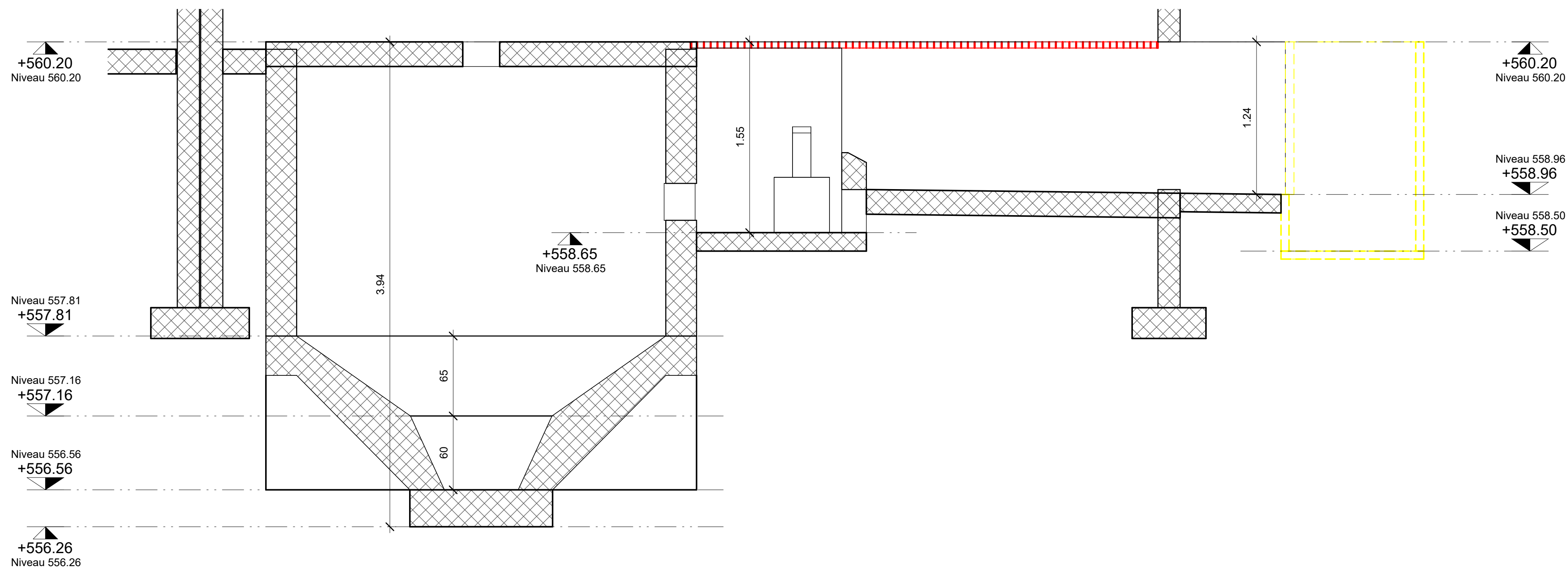
Coupe C - C 1 : 25
