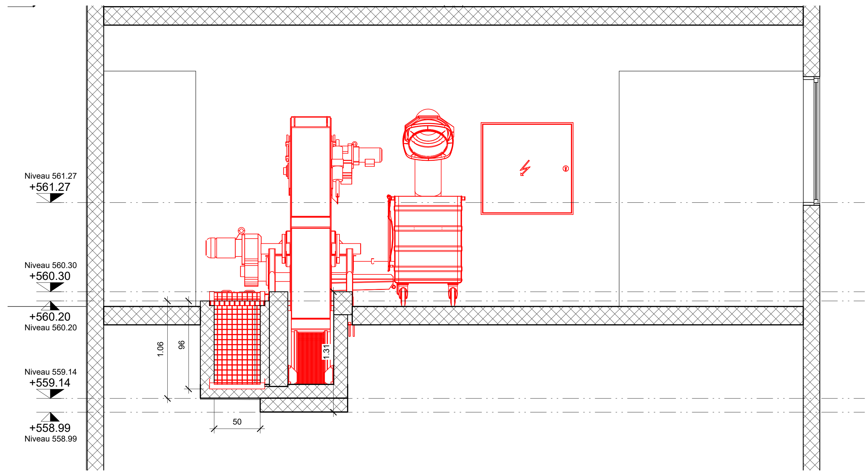
Coupe B - B 1 : 25
