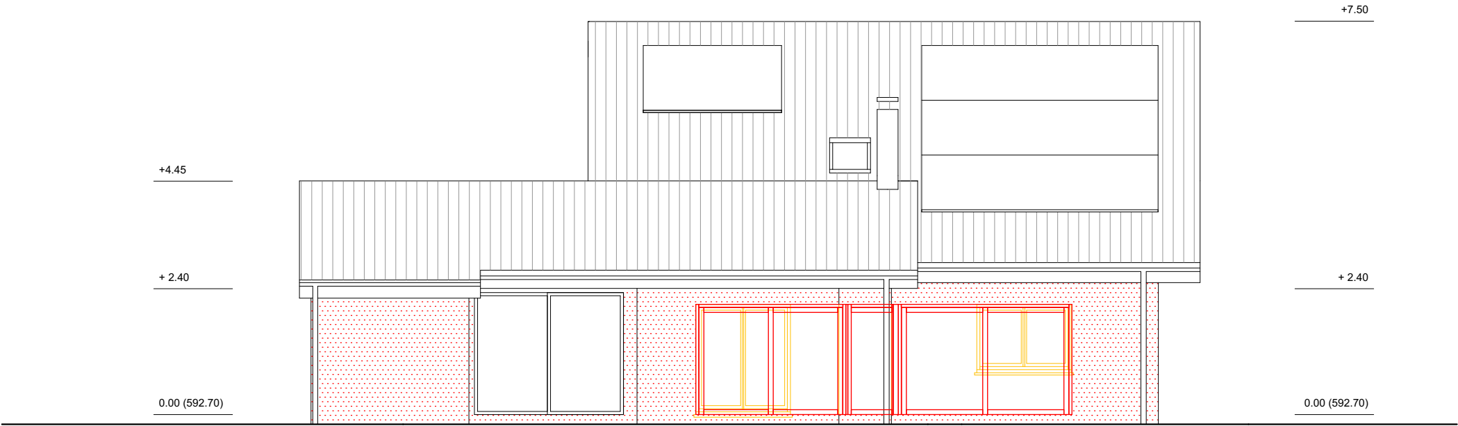
Élévation ouest
